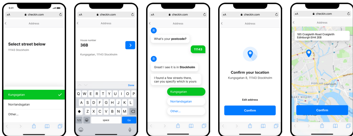
Grafik över några olika sätt som mjukvaran kan inhämta adressuppgifter från slutanvändaren.
